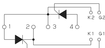
回路構成 Circuit Schema
