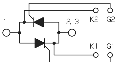
回路構成 Circuit Schema
