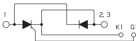
回路構成 Circuit Schema
