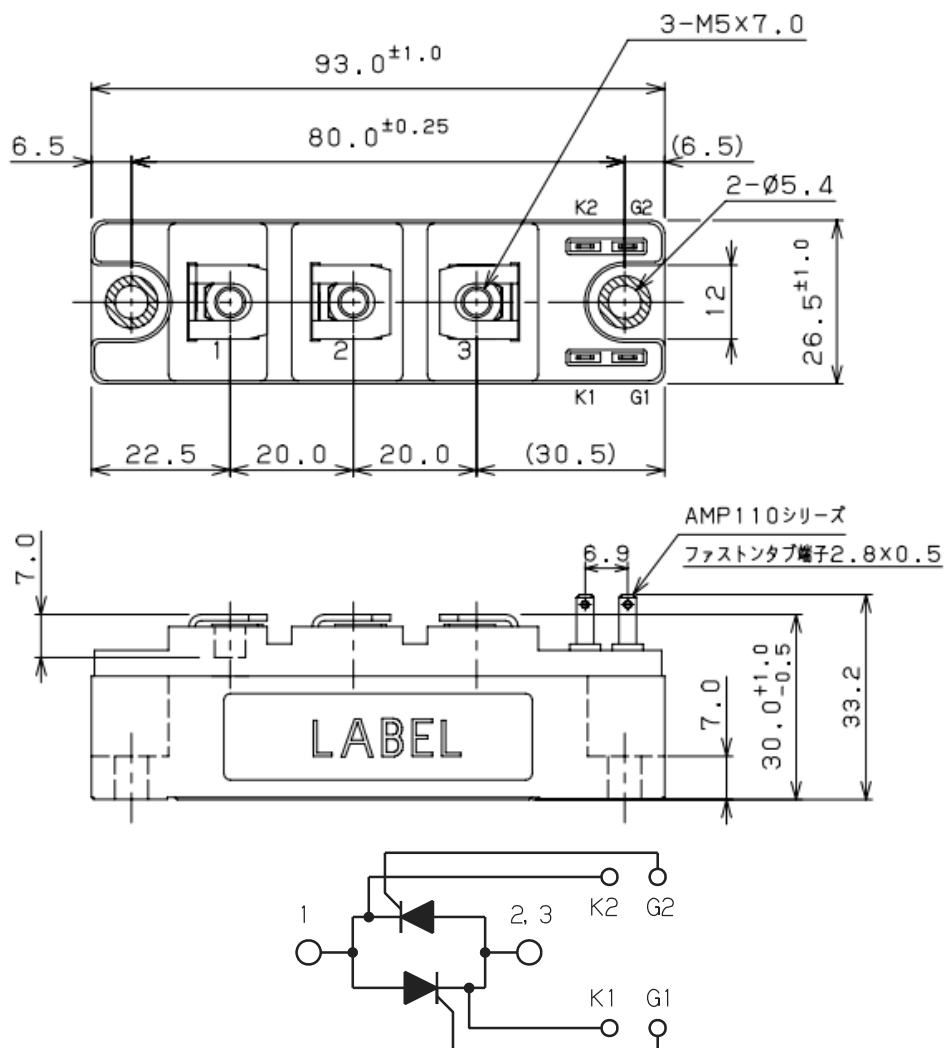
回路構成 Circuit Schema
